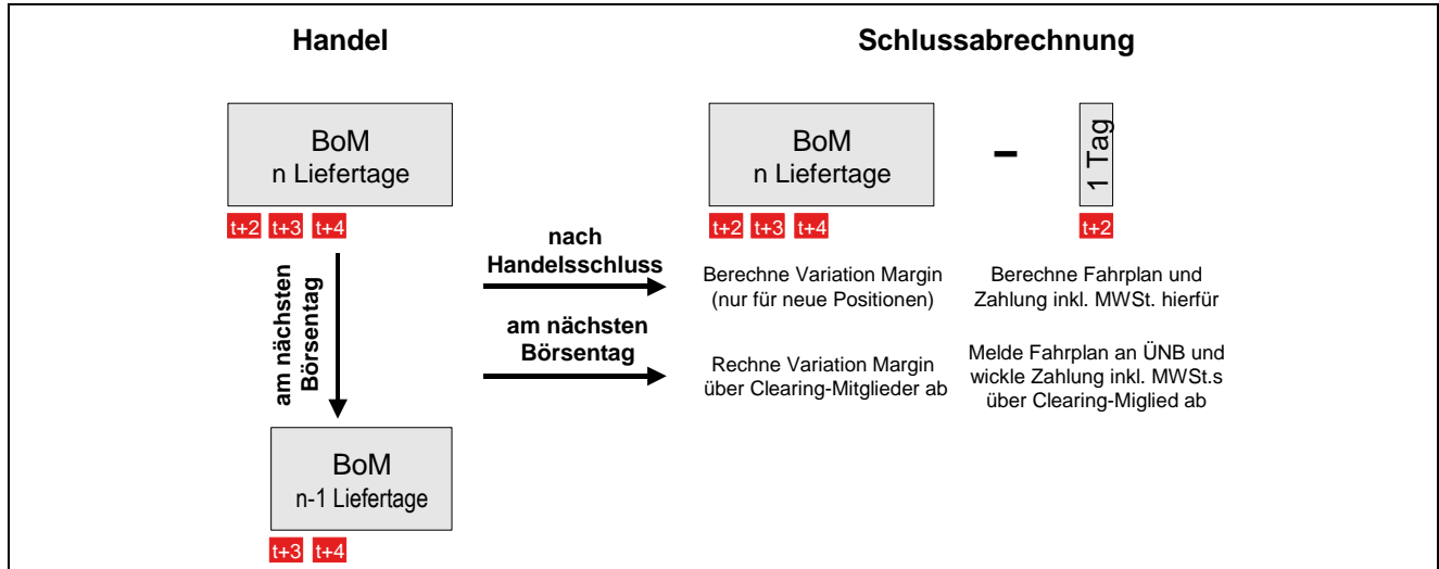
Abbildung 4.2: Physische Erfüllung von Baseload- und Peakload-Month-Futures
